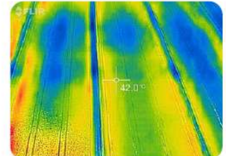
施工後：42.0°C
